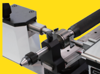
ねじプラグゲージの校正
