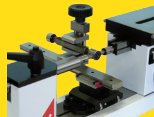
プラグゲージの校正
