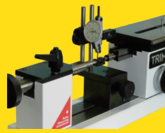
テストインジゲータの検査
