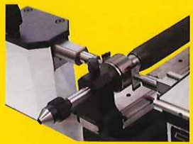
ねじプラグゲージの校正
