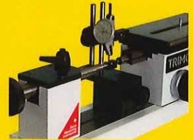
テストインジゲータの検査
