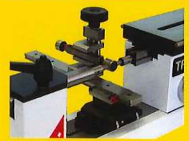
プラグゲージの校正
