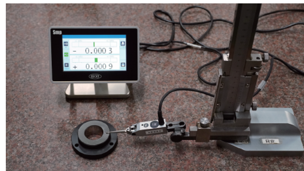
平行度測定（てこ式プローブ使用）
