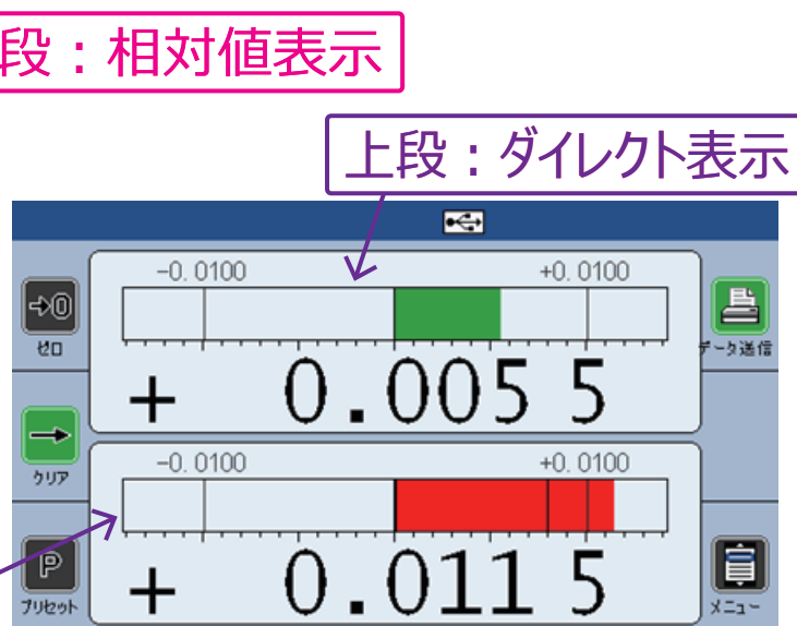
〔バーグラフ表示（中央）〕 （振れ測定）
